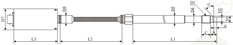
PT124系列外型尺寸图
