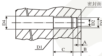
PT124系列 45°斜面密封安装孔尺寸图
