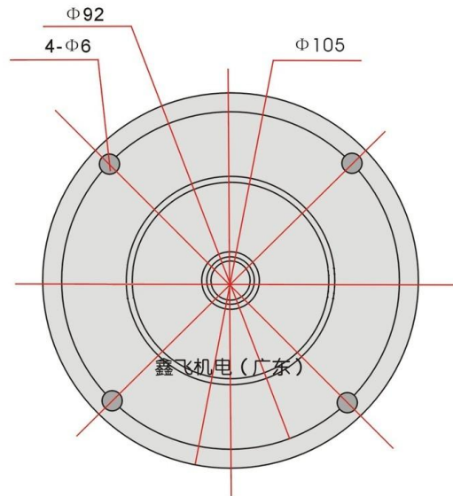
85CF测速机尺寸图
